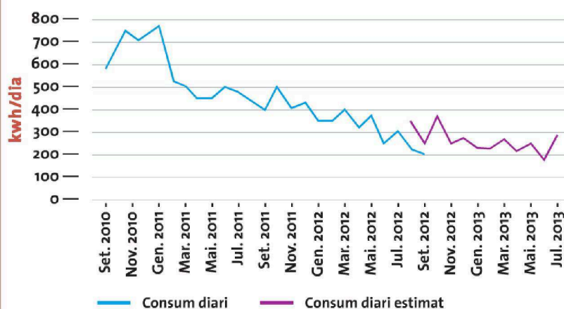
Evolució dels consums abans i després de la substitució de lluminàries el juliol de 2011. (Aparcament de Siracusa)
