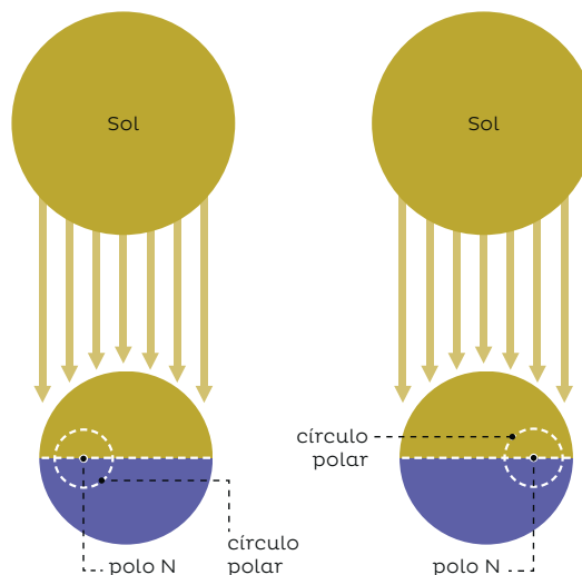
Figura 13. Iluminación de la Tierra durante los equinoccios vista desde el polo norte.
