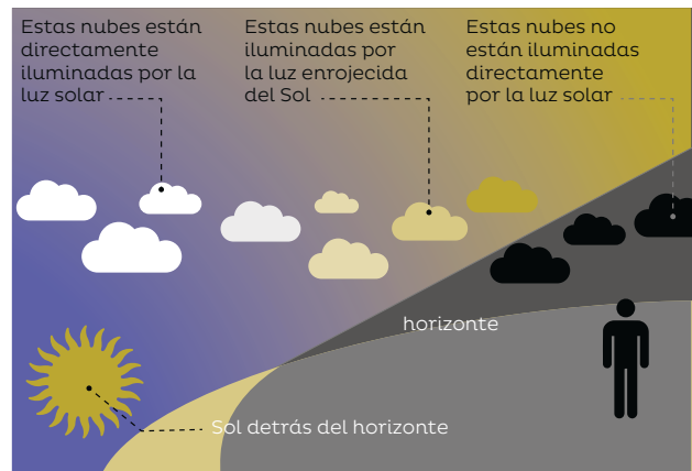
Figura 2. El color de la luz que ilumina las nubes determina su color.
