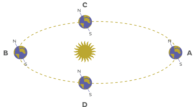
Figura 9. Movimiento de traslación de la Tierra en torno al Sol.
