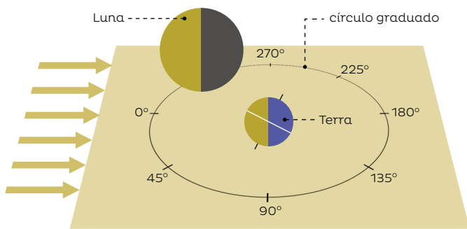
Figura 21. Maqueta para representar las fases de la Luna.
