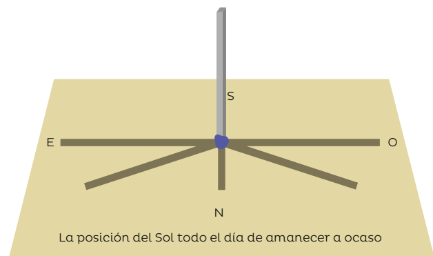
Figura 6. Las sombras se desplazan de oeste a este pasando por la dirección norte en el punto del mediodía. Las sombras a primera hora de la mañana y a última del atardecer son largas; el punto en el que son más cortas es en el de mediodía.
