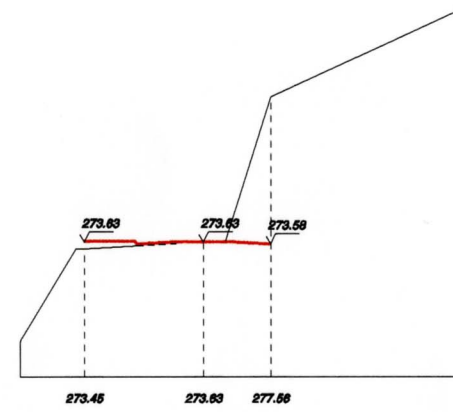
Cota +2.70 m. SECCIÓ CC'
