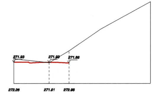
Cota +2.70 m. SECCIÓ DD'
