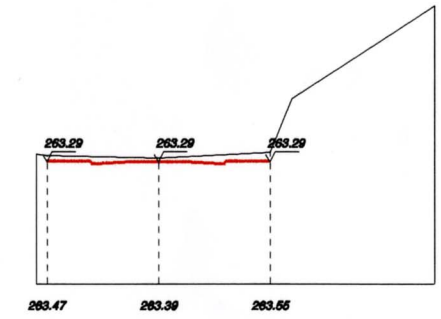
Cota +2.60 m. SECCIÓ HH'
