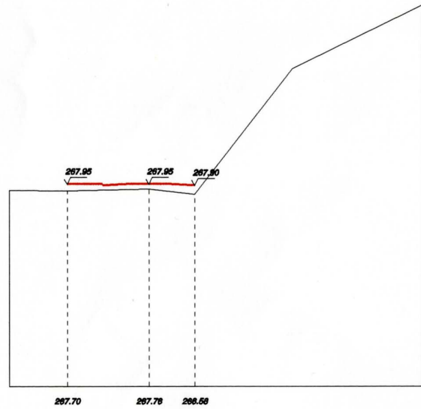
Cota +2.60 m. SECCIÓ EE'
