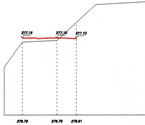
Cota +2.70 m. SECCIÓ BB'
