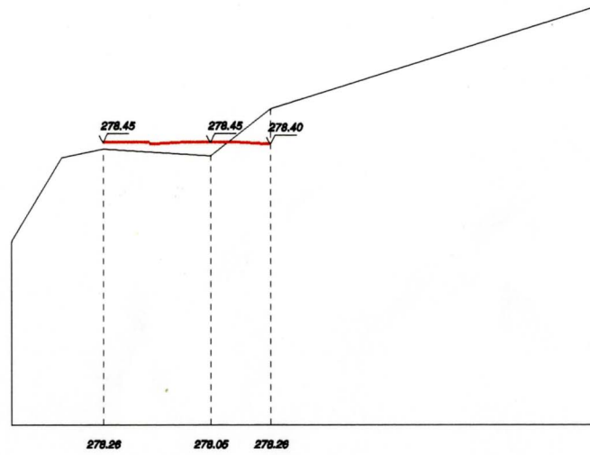
Cota +2.70 m. SECCIÓ AA'
