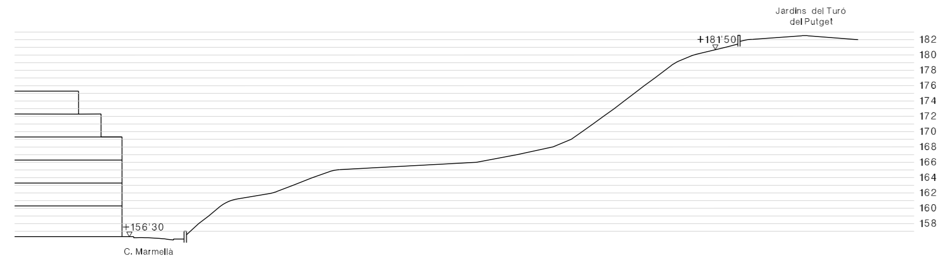
SECCIÓ B-B'
