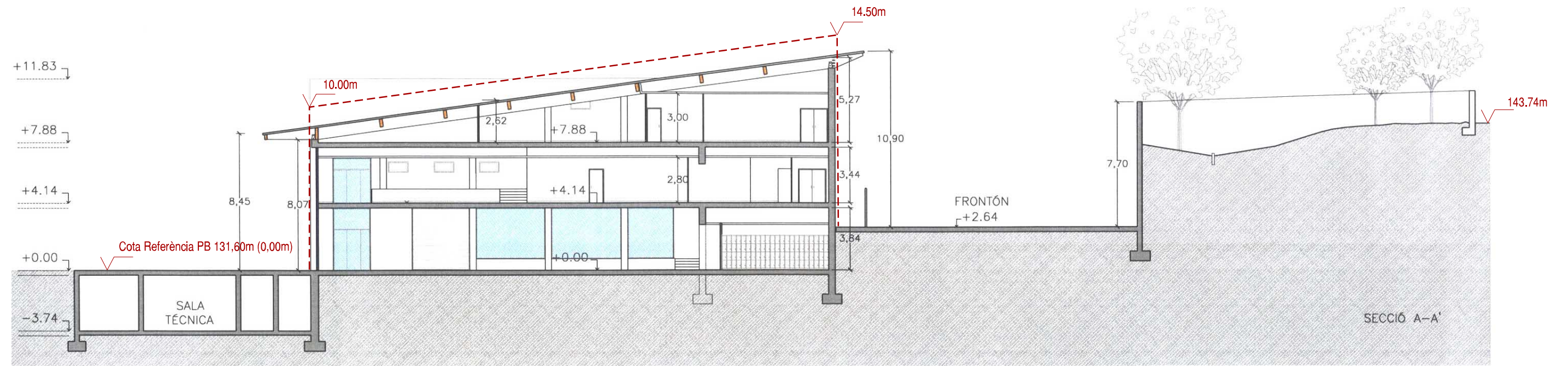
Secció AA'
