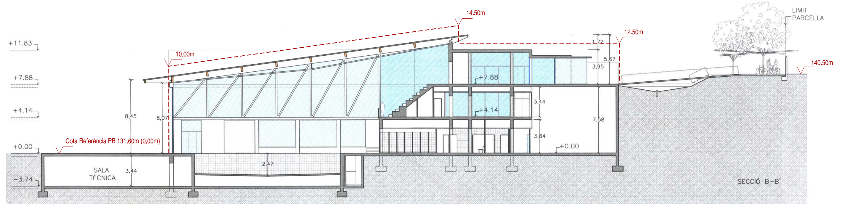
Secció BB'
