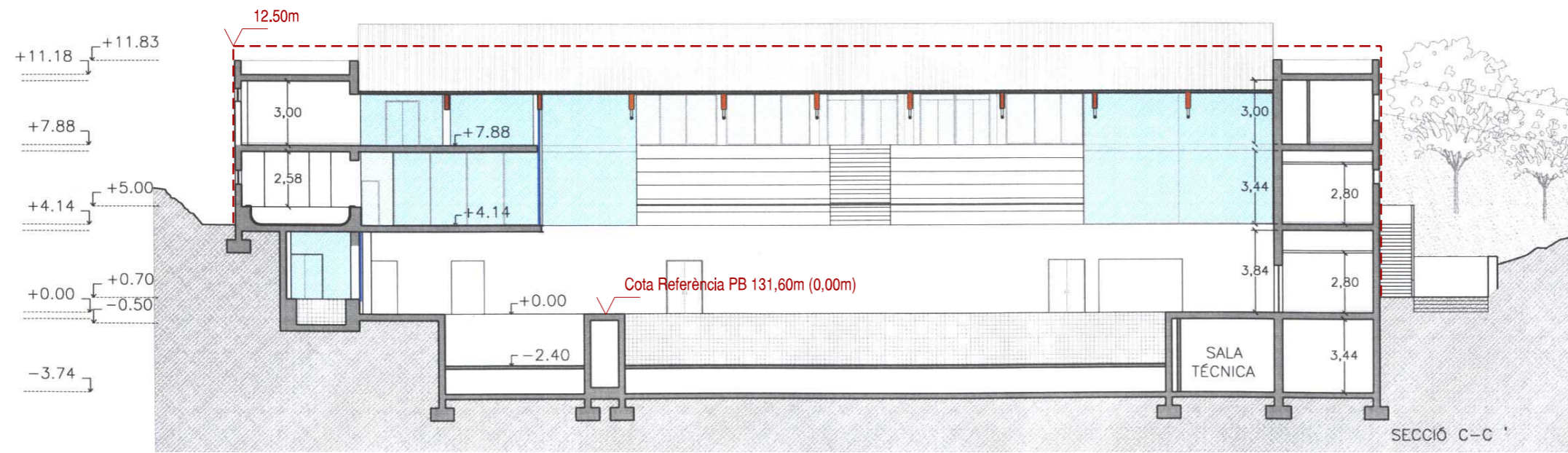
Secció CC'
