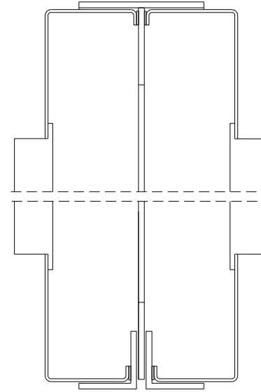
SECCIÓ A-A 1/ 2
