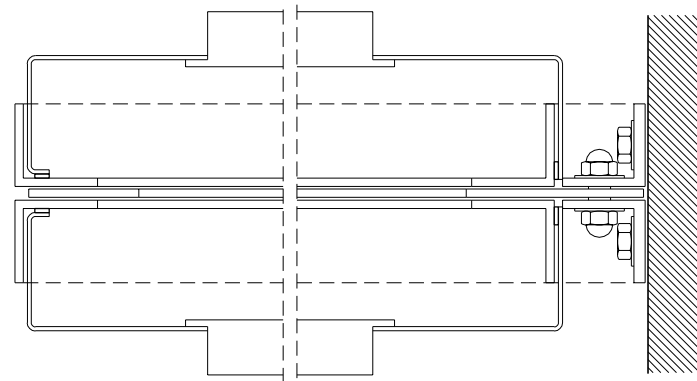
SECCIÓ B-B 1/ 2
