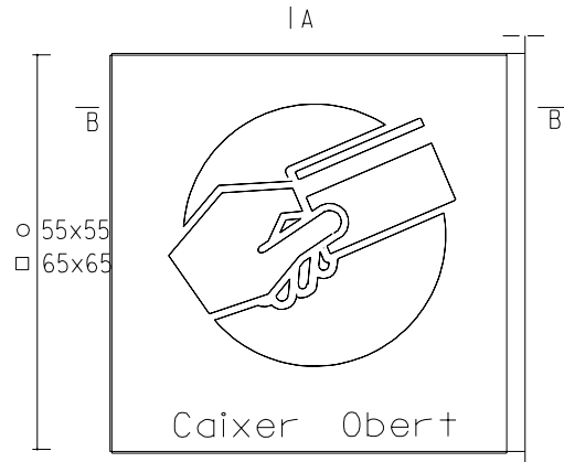
ALÇAT 1/10 | A
