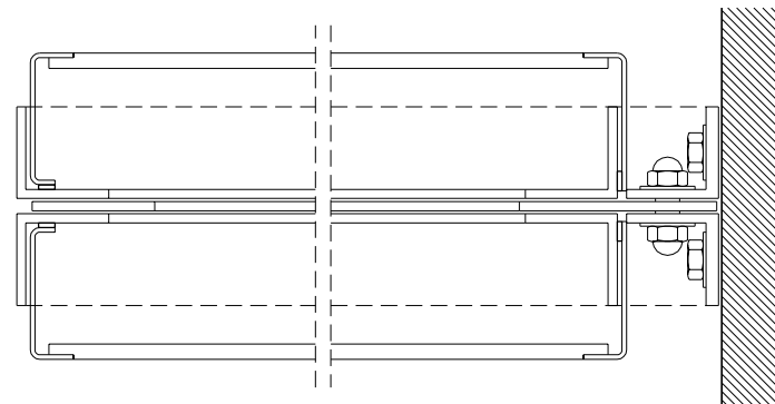
SECCIÓ B-B 1/2
