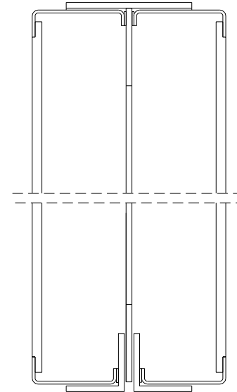
SECCIÓ A-A 1/2
