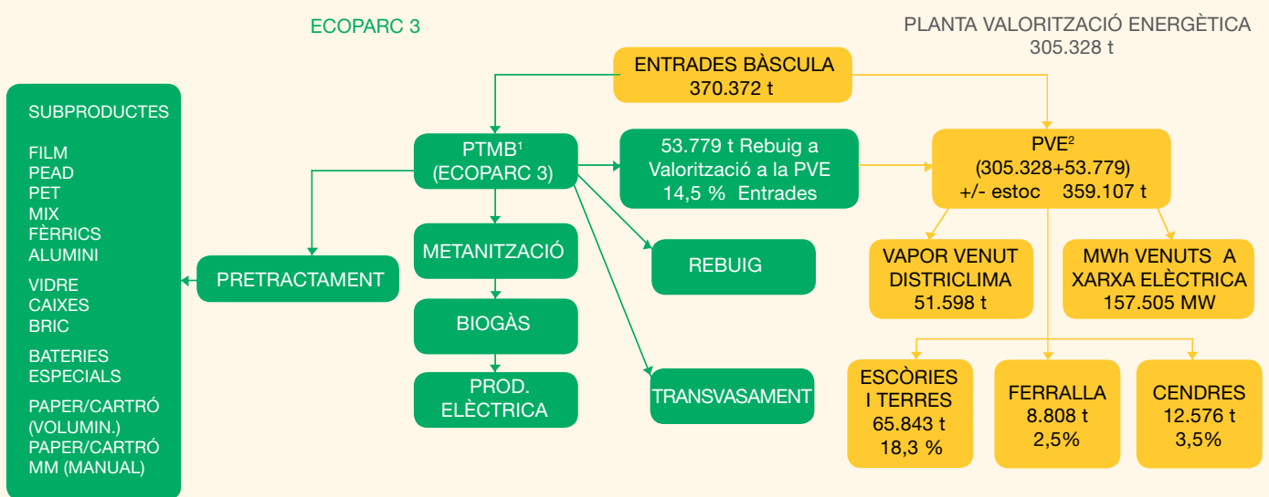
PVE: DIAGRAMA DE FLUXOS DE PRODUCCIÓ
