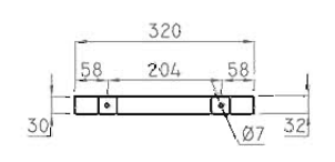
PLAFÓ ALUMINI
