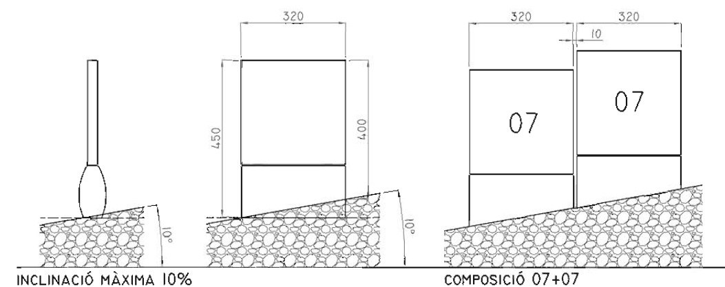
CONJUNTS I IMPLANTACIÓ EN PENDENT
