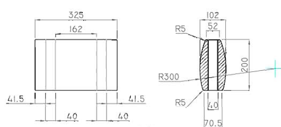
BASE DE FORMIGÓ
