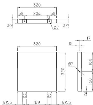
PLAFÓ ALUMINI
