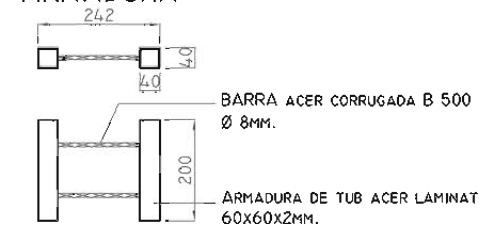
ARMADURA
