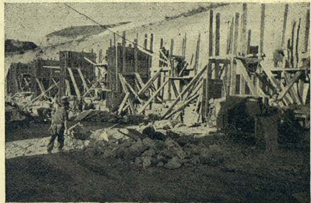
Fig. 8. — Detalle de los encofrados para la formación de muros para la construcción de grupos de nichos en el Cementerio del SO.
