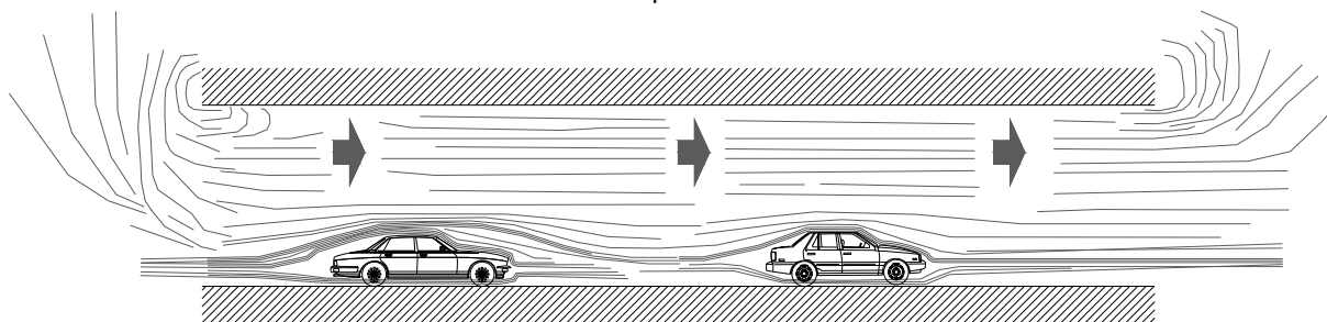
a) Inducció de cabal d'aire per efecte pistó
